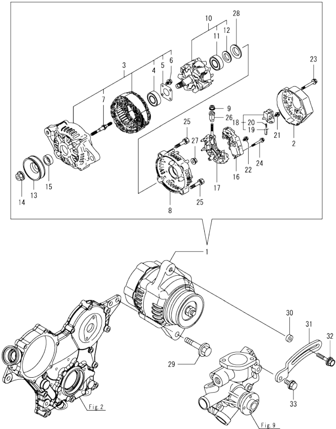
Fig.15. GENERATOR
